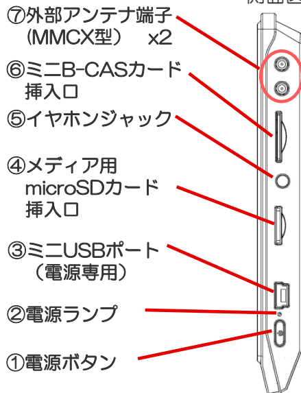
側面図
